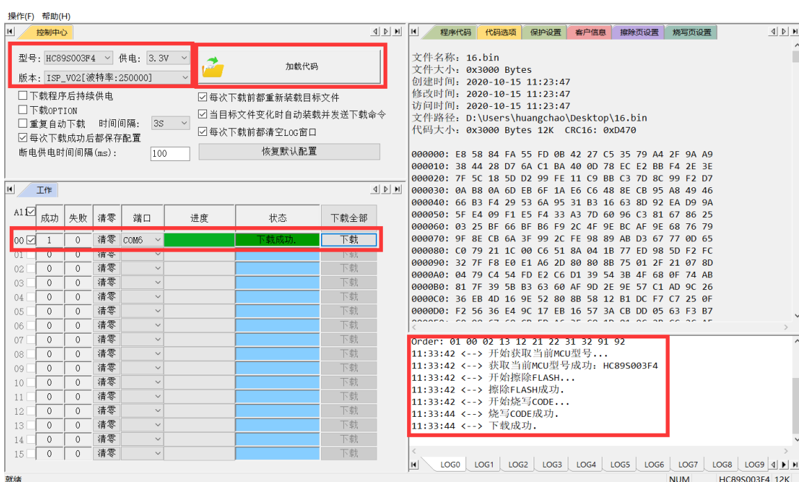
圖 2-3 連接 HC-LINK-V4 及支援 ISP_V02 的 HC89S003F4 晶片，
